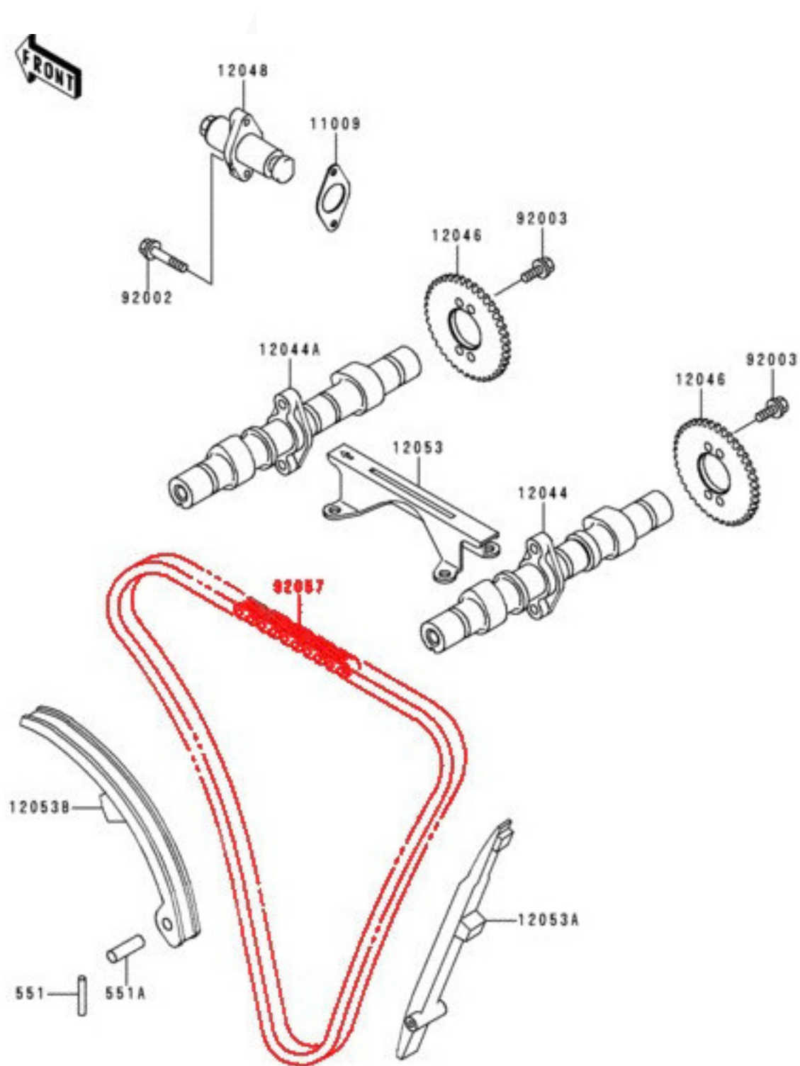
Schemat: Kawasaki KLE 500
