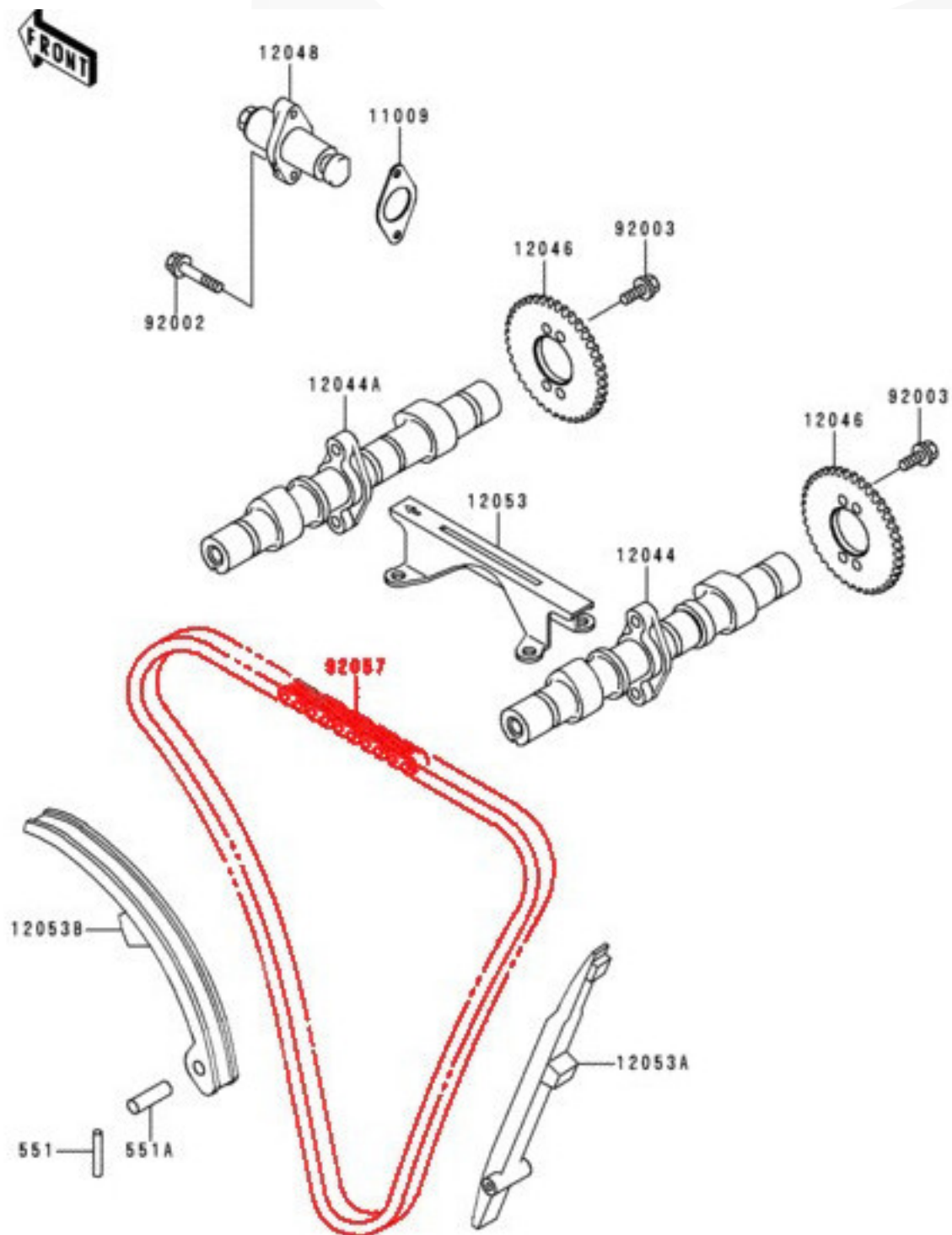
Schemat: Kawasaki KLE 500
